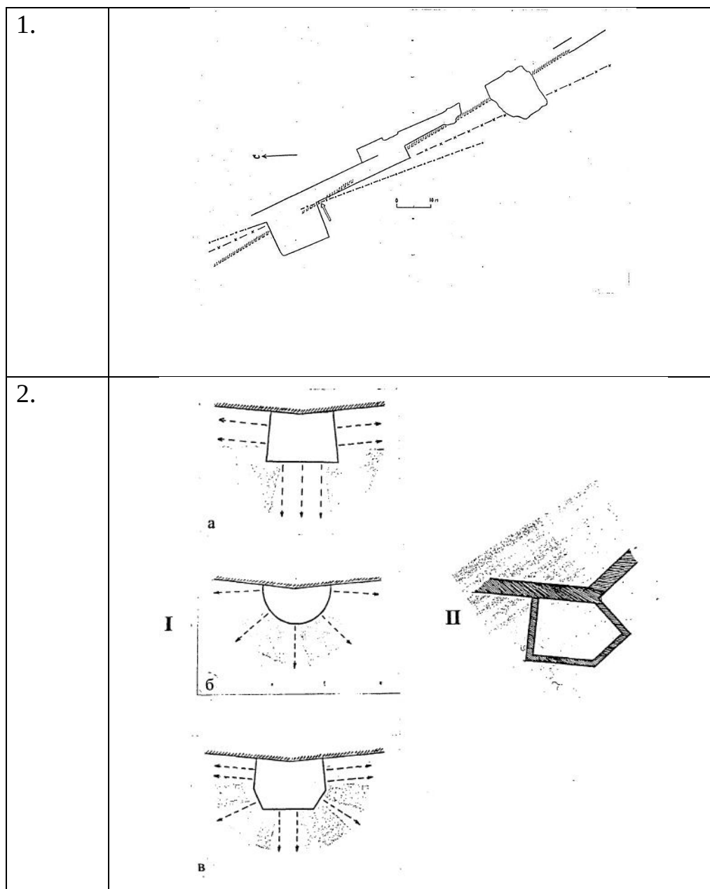
Рисунок 3.2.20. Возможные варианты планировочного решения эллинистических башен в комплексе «Западных ворот»:
