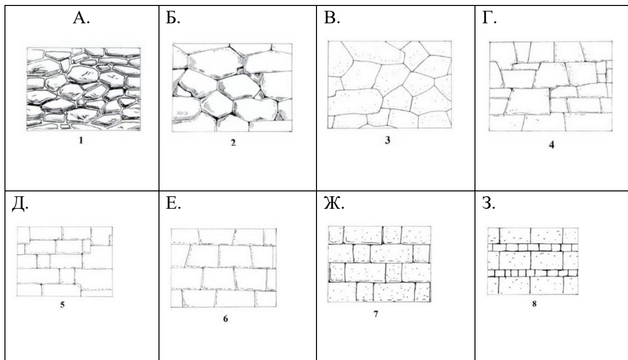
Рисунок 1.1. 28. Методы конструкций фортификационной архитектуры по Р. Скрапону.
