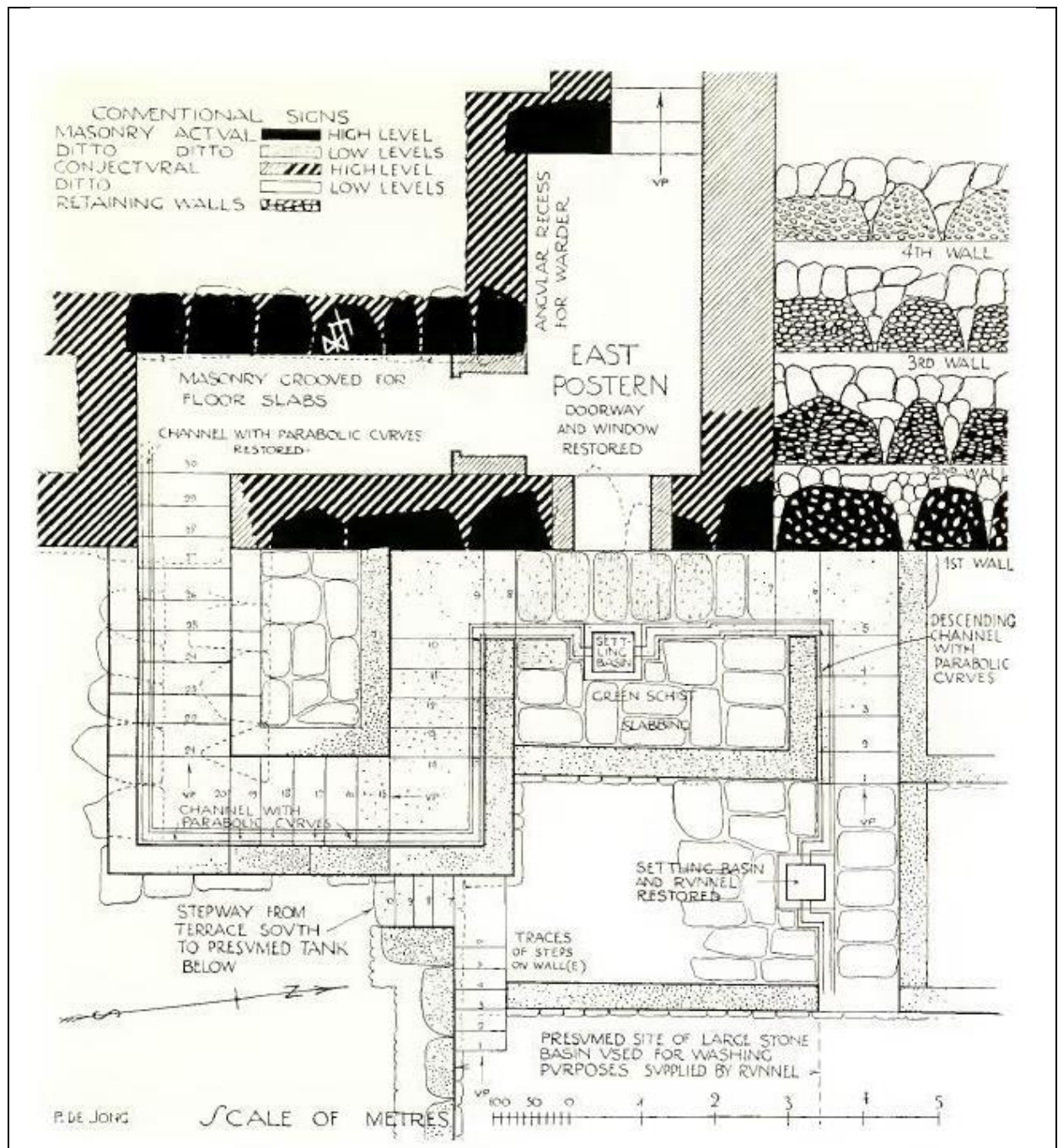
Рисунок 1.1.10. План Восточного бастиона и постерна.
