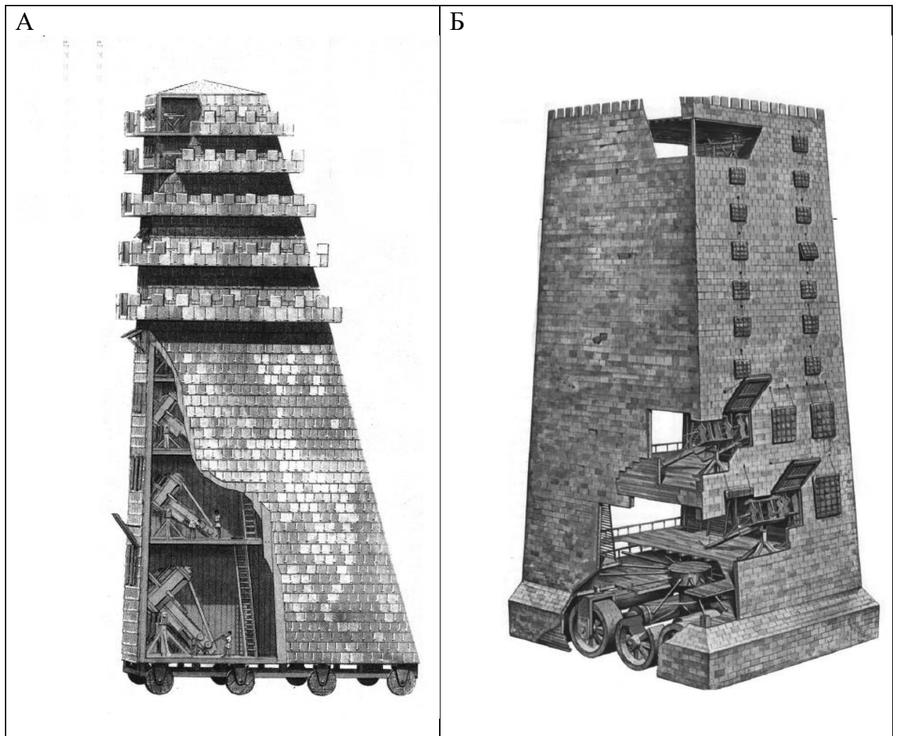
Рисунок 1.1.26. Графические реконструкция вариантов Гелеполы Деметрия Полиоркета. Архитектор Эпимах афинский.
