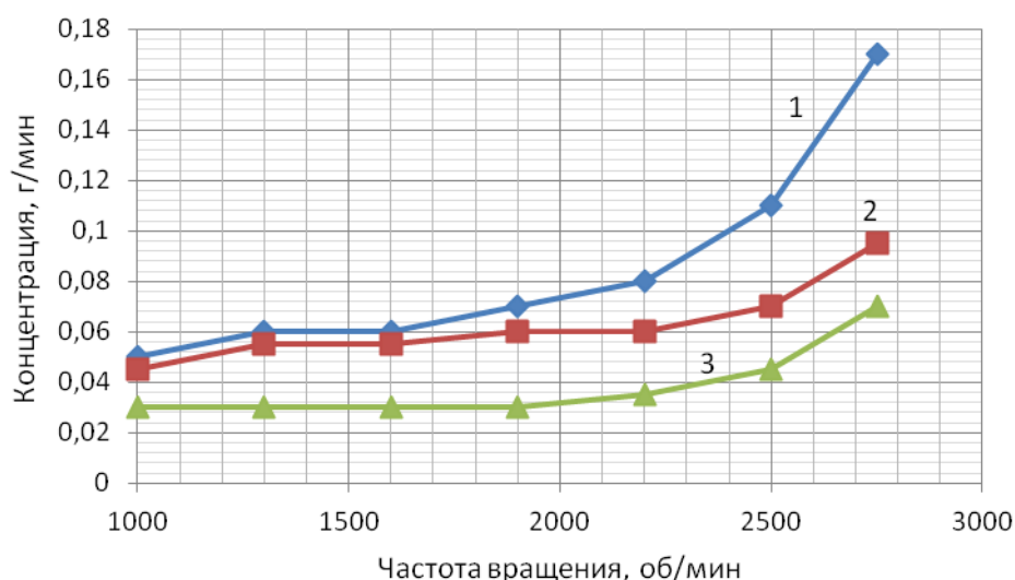
Рисунок 3.17 – Средние зависимости выбросов \text{NO}_x для двигателя Tector 4, установленного на автомобиле Iveco EuroCargo, мощностью 160 л.с. в режиме без нагрузки от оборотов коленчатого вала: 1 – базовая модель; 2 – при добавке 0,15% водорода к топливной смеси; 3 – при добавке 0,25% водорода к топливной смеси
