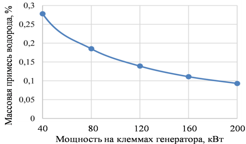
Рисунок 3.7 – Зависимость массовой примеси водорода \Delta H_2 от нагрузки ДВС специального автотранспорта
