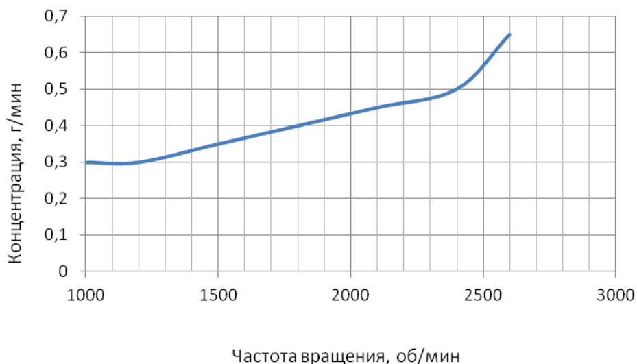
Рисунок 1.13 – Средняя зависимость выбросов CO от частоты вращения коленчатого вала двигателя Testor 4, мощностью 160 л.с., установленного на автомобиле Iveco EuroCargo в режиме нагрузки
