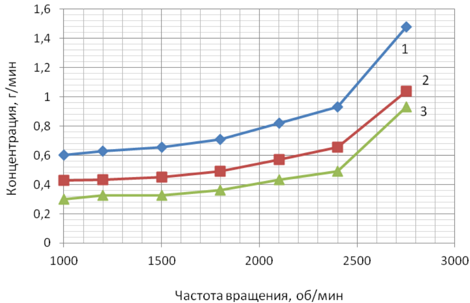
Рисунок 3.30 – Средние значения выбросов \text{SO}_2 для двигателя Tector 4, установленного на автомобиле Iveco EuroCargo, мощностью 180 л.с. в зависимости от частоты вращения коленчатого вала с нагрузкой: 1 – базовая модель; 2 – при добавке 0,15% водорода к топливной смеси; 3 – при добавке 0,25% водорода к топливной смеси
