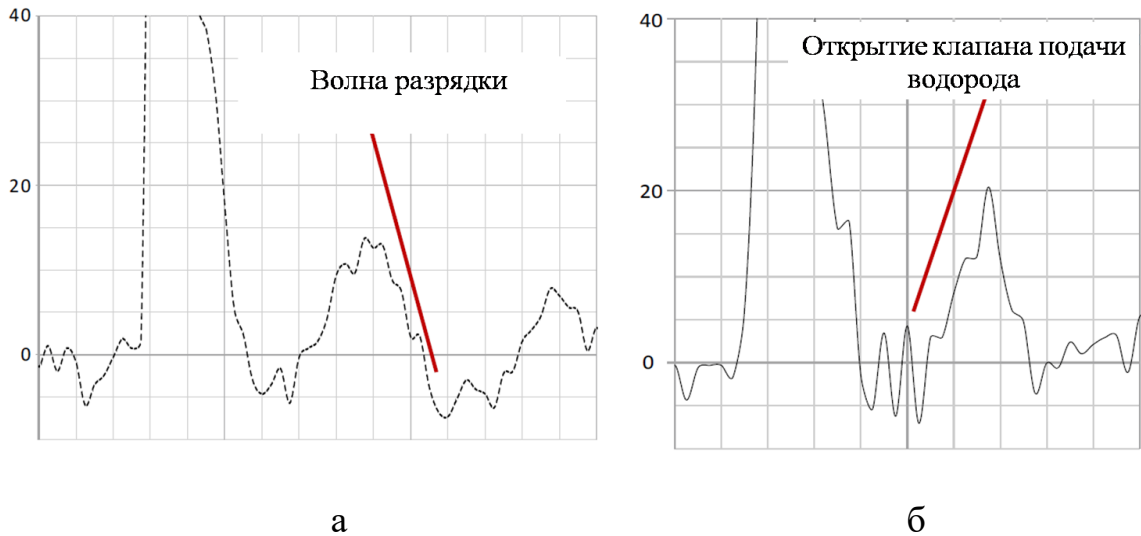
Рисунок 3.14 – Диаграммы давления водорода в топливопроводе высокого давления в ДВС спецавтотранспорта: а – без водорода; б – с водородом
