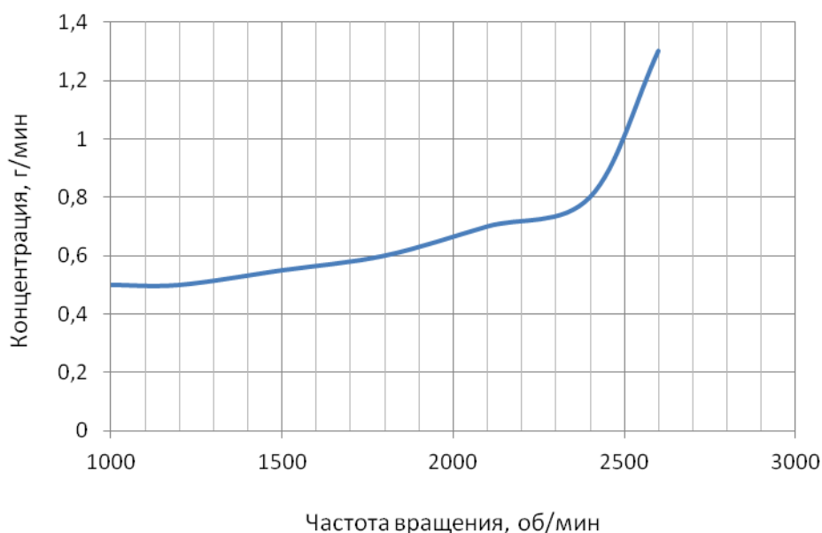
Рисунок 1.19 – Средние значения выбросов \text{SO}_2 для двигателя Tector 4, установленного на автомобиле Iveco EuroCargo, мощностью 160 л.с. в зависимости от частоты вращения коленчатого вала с нагрузкой
