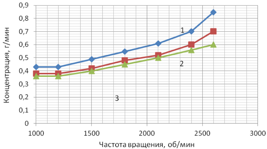
Рисунок 3.40 – Средние зависимости выбросов CO от частоты вращения коленчатого вала двигателя Tector 6, мощностью 280 л.с., установленного на автомобиле Iveco EuroCargo в режиме нагрузки: 1 – базовая модель; 2 – при добавке 0,15% водорода к топливной смеси; 3 – при добавке 0,25% водорода к топливной смеси
