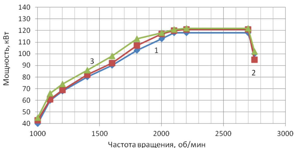
Рисунок 3.5 – Зависимости средней эффективной мощности от частоты вращения коленчатого вала двигателя Testor 4, мощностью 160 л.с.: 1 – базовая модель; 2 – при добавке 0,15% водорода к топливной смеси; 3 – при добавке 0,25% водорода к топливной смеси
