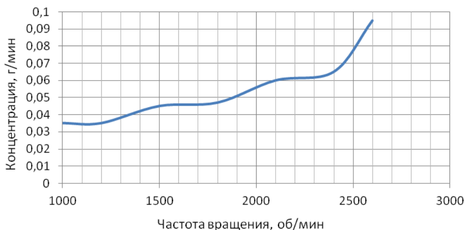
Рисунок 1.17 – Зависимость средних значений выбросов НС для двигателя Testor 4, установленного на автомобиле Iveco EuroCargo, мощностью 160 л.с. под нагрузкой от частоты вращения коленчатого вала
