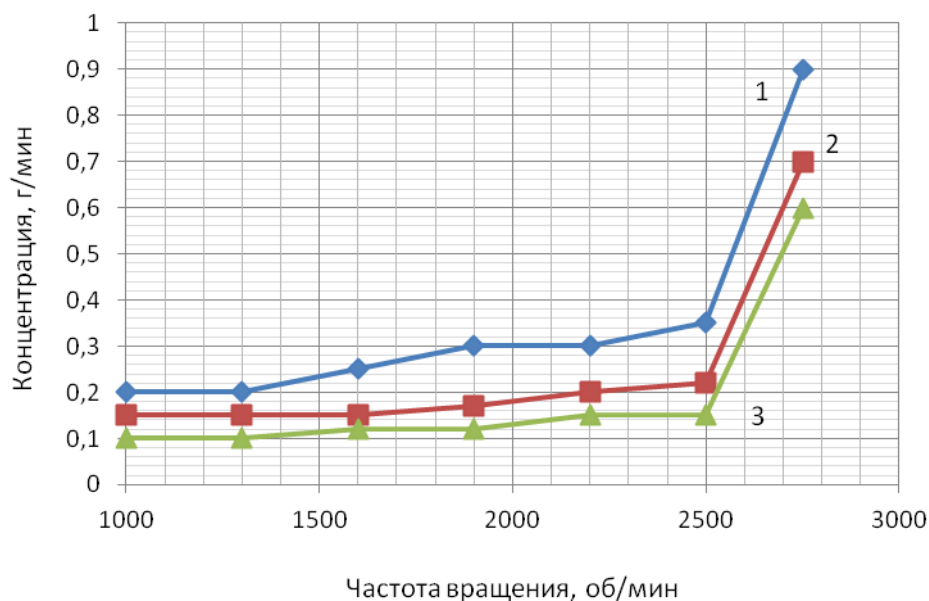
Рисунок 3.15 – Средние зависимости выбросов СО для двигателя Tector 4, установленного на автомобиле Iveco EuroCargo, мощностью 160 л.с. от частоты вращения коленчатого вала в режиме без нагрузки: 1 – базовая модель; 2 – при добавке 0,15% водорода к топливной смеси; 3 – при добавке 0,25% водорода к топливной смеси
