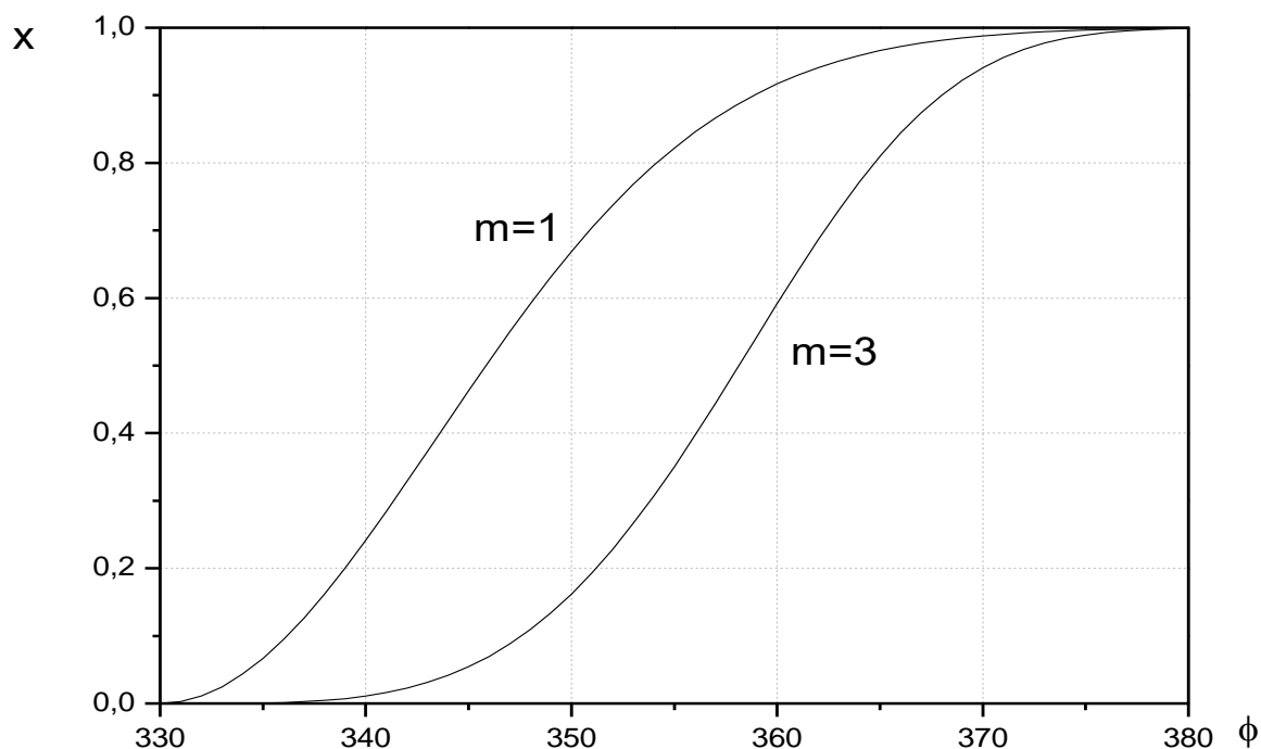
Рисунок 2.2 – Полученный закон сгорания для ДВС, работающего по смешанному циклу дизеля и примесей водорода
