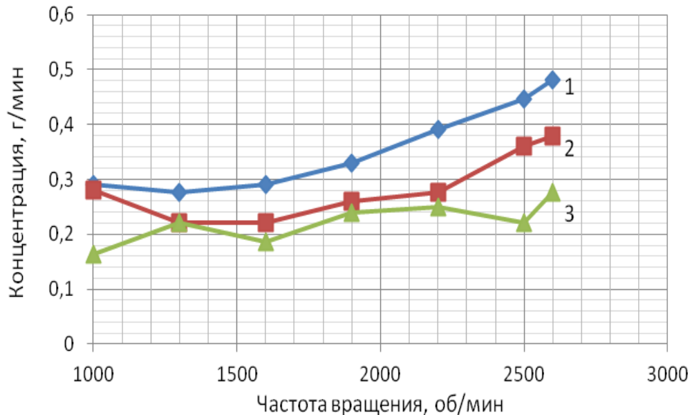
Рисунок 3.31 – Средние зависимости выбросов СО для двигателя Tector 6, установленного на автомобиле Iveco EuroCargo, мощностью 220 л.с. от частоты вращения коленчатого вала в режиме без нагрузки: 1 – базовая модель; 2 – при добавке 0,15% водорода к топливной смеси; 3 – при добавке 0,25% водорода к топливной смеси
