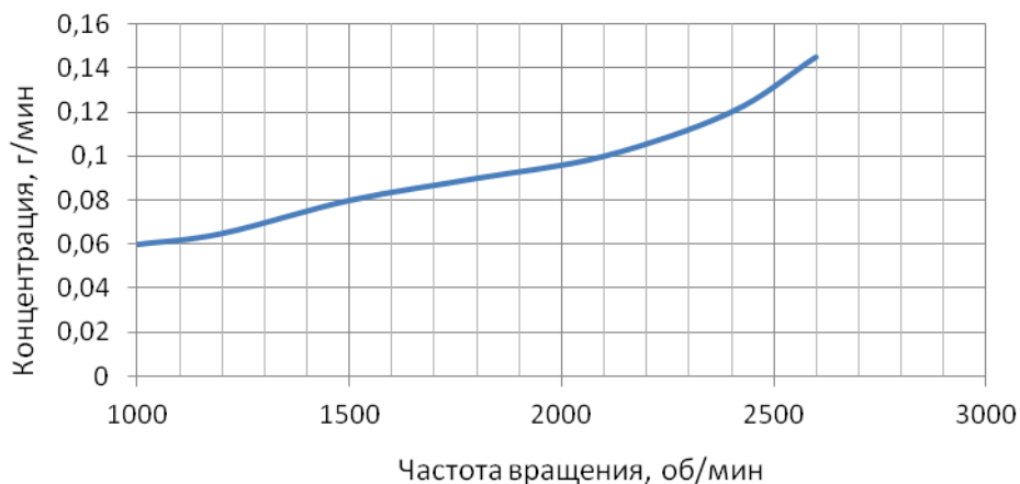
Рисунок 1.14 – Средние зависимости выбросов NO x для двигателя Testor 6, установленного на автомобиле Iveco EuroCargo, мощностью 220 л.с. в режиме без нагрузки от оборотов коленчатого вала
