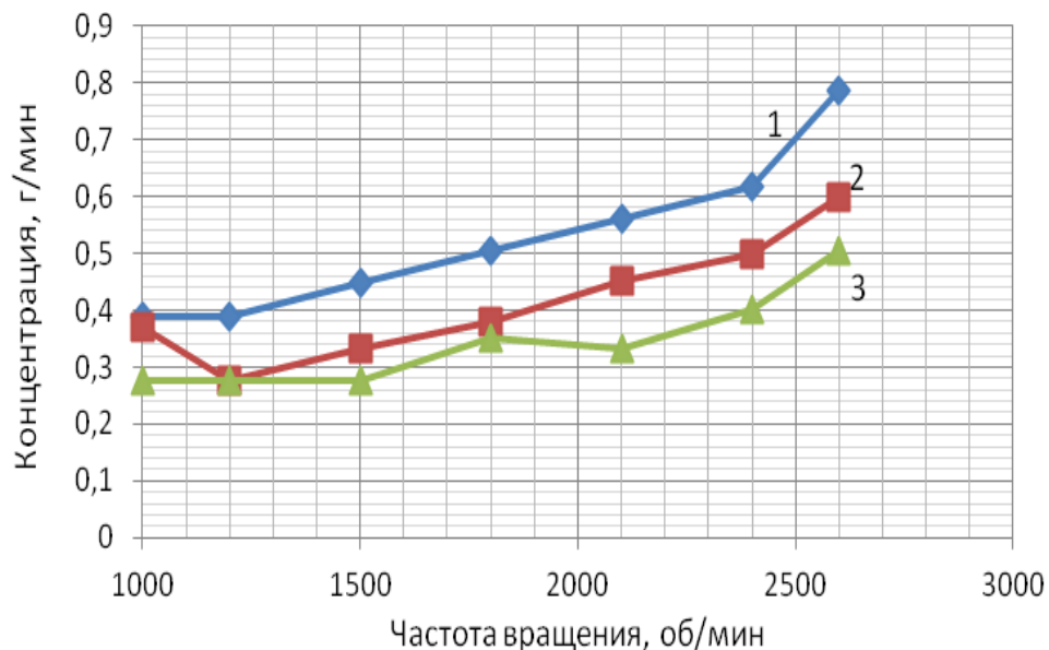
Рисунок 3.32 – Средние зависимости выбросов СО от частоты вращения коленчатого вала двигателя Tector 6, мощностью 220 л.с., установленного на автомобиле Iveco EuroCargo в режиме нагрузки: 1 – базовая модель; 2 – при добавке 0,15% водорода к топливной смеси; 3 – при добавке 0,25% водорода к топливной смеси
