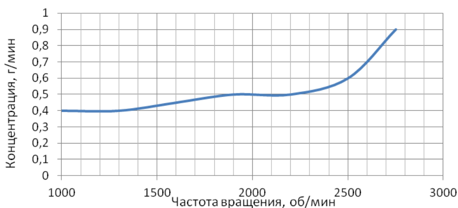
Рисунок 1.18 – Зависимости средних значений выбросов SO_2 для двигателя Testor 4, установленного на автомобиле Iveco EuroCargo, мощностью 160 л.с. без нагрузки от частоты вращения коленчатого вала
