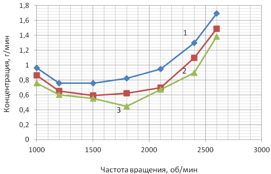
Рисунок 3.46 – Средние значения выбросов \text{SO}_2 для двигателя Tector 6, установленного на автомобиле Iveco EuroCargo, мощностью 280 л.с. в зависимости от частоты вращения коленчатого вала с нагрузкой: 1 – базовая модель; 2 – при добавке 0,15% водорода к топливной смеси; 3 – при добавке 0,25% водорода к топливной смеси
