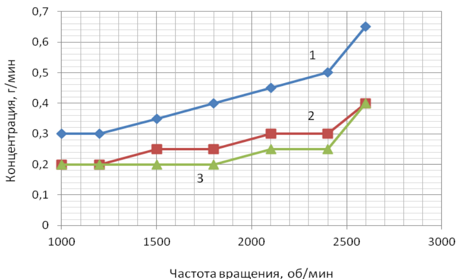
Рисунок 3.16 – Средние зависимости выбросов СО от частоты вращения коленчатого вала двигателя Tector 4, мощностью 160 л.с., установленного на автомобиле Iveco EuroCargo в режиме нагрузки: 1 – базовая модель; 2 – при добавке 0,15% водорода к топливной смеси; 3 – при добавке 0,25% водорода к топливной смеси
