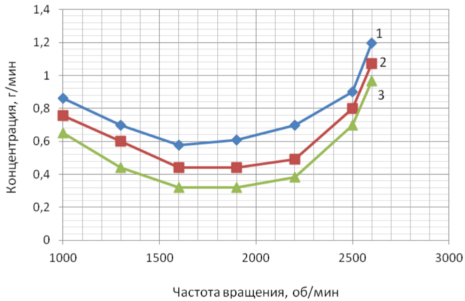
Рисунок 3.45 – Зависимости средних значений выбросов \text{SO}_2 для двигателя Tector 6, установленного на автомобиле Iveco EuroCargo, мощностью 280 л.с. без нагрузки от частоты вращения коленчатого вала: 1 – базовая модель; 2 – при добавке 0,15% водорода к топливной смеси; 3 – при добавке 0,25% водорода к топливной смеси
