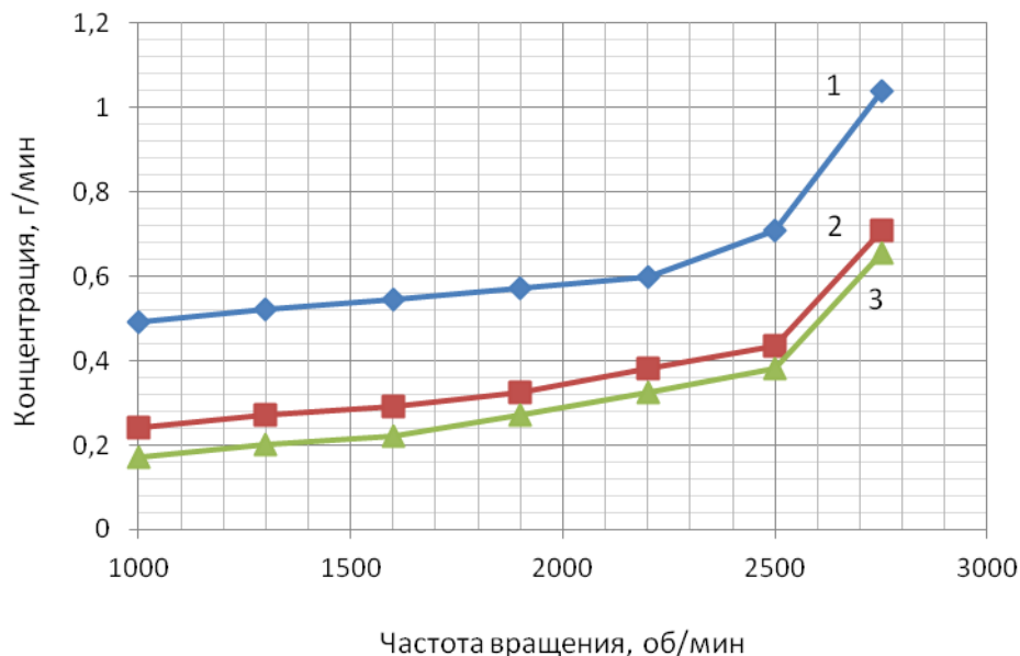
Рисунок 3.29 – Зависимости средних значений выбросов SO_2 для двигателя Tector 4, установленного на автомобиле Iveco EuroCargo, мощностью 180 л.с. без нагрузки от частоты вращения коленчатого вала: 1 – базовая модель; 2 – при добавке 0,15% водорода к топливной смеси; 3 – при добавке 0,25% водорода к топливной смеси
