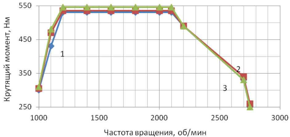
Рисунок 3.6 – Зависимости среднего крутящего момента от частоты вращения коленчатого вала двигателя Tector 4, мощностью 160 л.с.: 1 – базовая модель; 2 – при добавке 0,15% водорода к топливной смеси; 3 – при добавке 0,25% водорода к топливной смеси
