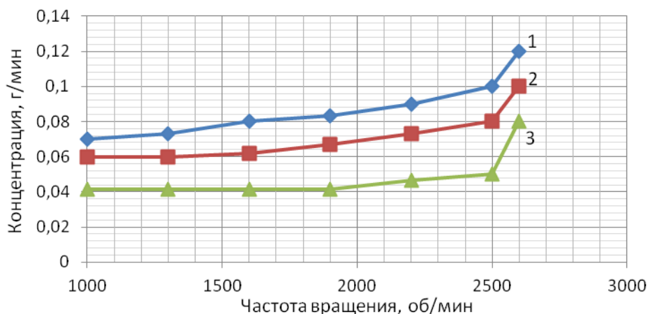
Рисунок 3.25 – Средние зависимости выбросов \text{NO}_x для двигателя Tector 4, установленного на автомобиле Iveco EuroCargo, мощностью 180 л.с. в режиме без нагрузки от оборотов коленчатого вала: 1 – базовая модель; 2 – при добавке 0,15% водорода к топливной смеси; 3 – при добавке 0,25% водорода к топливной смеси
