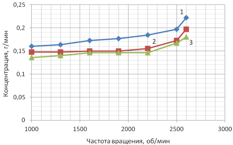
Рисунок 3.41 – Средние зависимости выбросов \text{NO}_x для двигателя Tector 6, установленного на автомобиле Iveco EuroCargo, мощностью 280 л.с. в режиме без нагрузки от оборотов коленчатого вала: 1 – базовая модель; 2 – при добавке 0,15% водорода к топливной смеси; 3 – при добавке 0,25% водорода к топливной смеси
