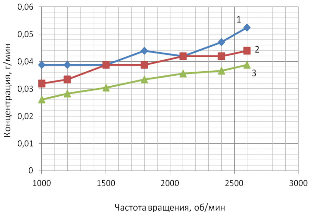
Рисунок 3.28 – Зависимости средних значений выбросов НС для двигателя Tector 4, установленного на автомобиле Iveco EuroCargo, мощностью 180 л.с. под нагрузкой от частоты вращения коленчатого вала: 1 – базовая модель; 2 – при добавке 0,15% водорода к топливной смеси; 3 – при добавке 0,25% водорода к топливной смеси
