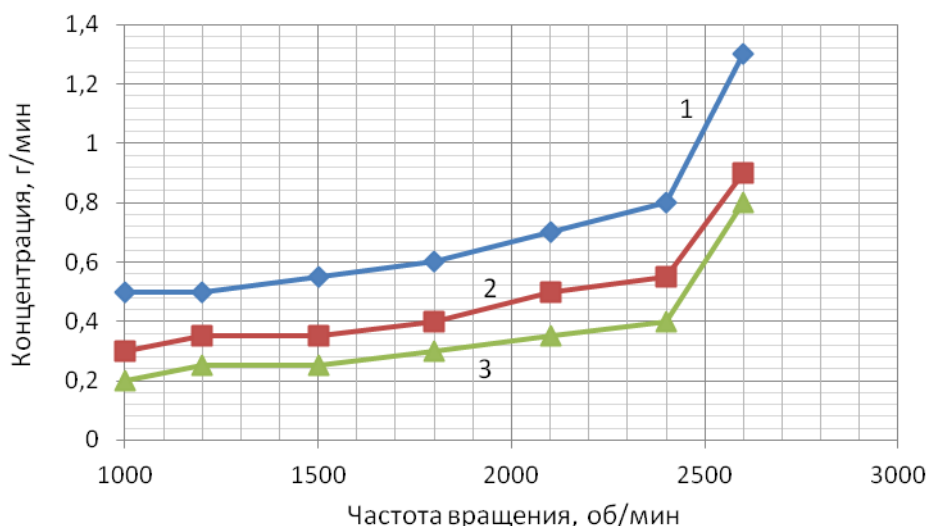
Рисунок 3.22 – Средние значения выбросов \text{SO}_2 для двигателя Tector 4, установленного на автомобиле Iveco EuroCargo, мощностью 160 л.с. в зависимости от частоты вращения коленчатого вала с нагрузкой: 1 – базовая модель; 2 – при добавке 0,15% водорода к топливной смеси; 3 – при добавке 0,25% водорода к топливной смеси
