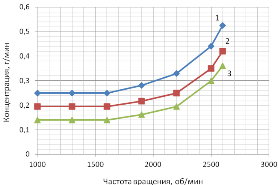
Рисунок 3.23 – Средние зависимости выбросов CO для двигателя Testor 4, установленного на автомобиле Iveco EuroCargo, мощностью 180 л.с. от частоты вращения коленчатого вала в режиме без нагрузки: 1 – базовая модель; 2 – при добавке 0,15% водорода к топливной смеси; 3 – при добавке 0,25% водорода к топливной смеси
