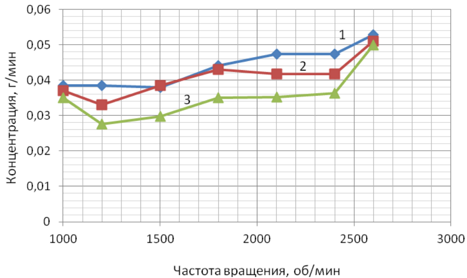
Рисунок 3.36 – Зависимости средних значений выбросов HC для двигателя Testor 6, установленного на автомобиле Iveco EuroCargo, мощностью 220 л.с. под нагрузкой от частоты вращения коленчатого вала: 1 – базовая модель; 2 – при добавке 0,15% водорода к топливной смеси; 3 – при добавке 0,25% водорода к топливной смеси
