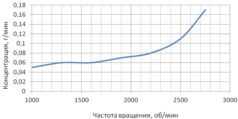
Рисунок 1.14 – Средние зависимости выбросов NO x для двигателя Testor 6, установленного на автомобиле Iveco EuroCargo, мощностью 220 л.с. в режиме без нагрузки от оборотов коленчатого вала
