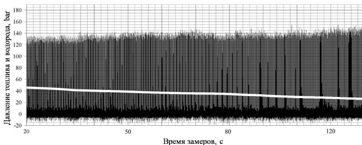
Рисунок 3.13 – График зависимости максимального давления впрыска топливо-водородной смеси от давления водорода в ДВС специального автотранспорта
