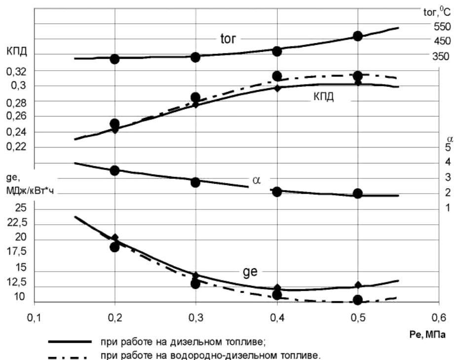
Рисунок 1.20 – Нагрузочная характеристика дизельного двигателя
