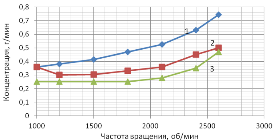
Рисунок 3.24 – Средние зависимости выбросов СО от частоты вращения коленчатого вала двигателя Tector 4, мощностью 180 л.с., установленного на автомобиле Iveco EuroCargo в режиме нагрузки: 1 – базовая модель; 2 – при добавке 0,15% водорода к топливной смеси; 3 – при добавке 0,25% водорода к топливной смеси
