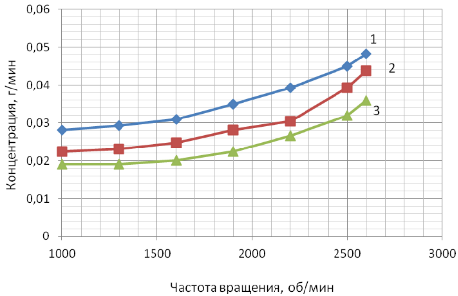
Рисунок 3.43 – Зависимости средних значений выбросов HC для двигателя Tector 6, установленного на автомобиле Iveco Euro Cargo, мощностью 280 л.с. в режиме без нагрузки от частоты вращения коленчатого вала: 1 – базовая модель; 2 – при добавке 0,15% водорода к топливной смеси; 3 – при добавке 0,25% водорода к топливной смеси
