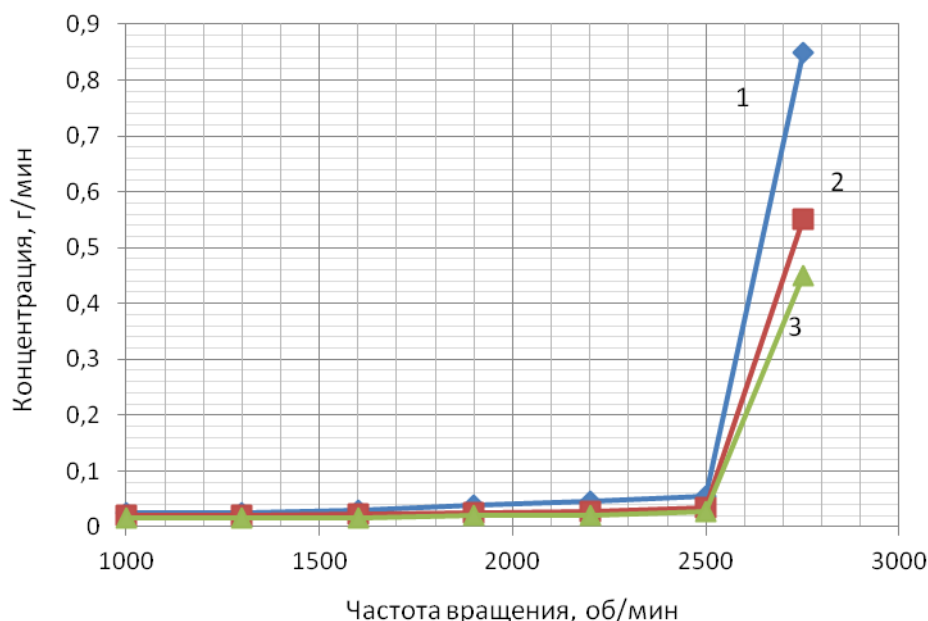
Рисунок 3.19 – Зависимости средних значений выбросов НС для двигателя Tector 4, установленного на автомобиле Iveco EuroCargo, мощностью 160 л.с. в режиме без нагрузки от частоты вращения коленчатого вала: 1 – базовая модель; 2 – при добавке 0,15% водорода к топливной смеси; 3 – при добавке 0,25% водорода к топливной смеси
