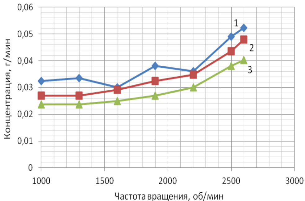
Рисунок 3.27 – Зависимости средних значений выбросов НС для двигателя Testor 4, установленного на автомобиле Iveco EuroCargo, мощностью 180 л.с. в режиме без нагрузки от частоты вращения коленчатого вала: 1 – базовая модель; 2 – при добавке 0,15% водорода к топливной смеси; 3 – при добавке 0,25% водорода к топливной смеси
