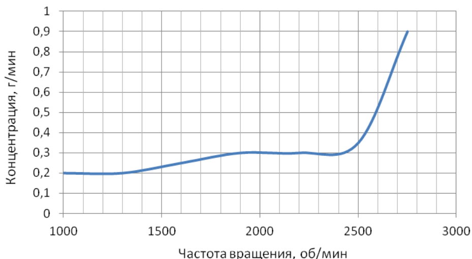
Рисунок 1.12 – Средняя зависимость выбросов CO для двигателя Testor 4, установленного на автомобиле Iveco EuroCargo, мощностью 160 л.с. от частоты вращения коленчатого вала в режиме без нагрузки
