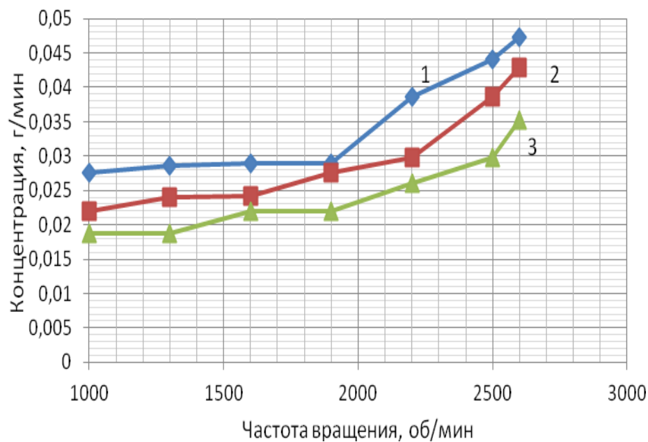
Рисунок 3.35 – Зависимости средних значений выбросов НС для двигателя Tector 6, установленного на автомобиле Iveco EuroCargo, мощностью 220 л.с. в режиме без нагрузки от частоты вращения коленчатого вала: 1 – базовая модель; 2 – при добавке 0,15% водорода к топливной смеси; 3 – при добавке 0,25% водорода к топливной смеси
