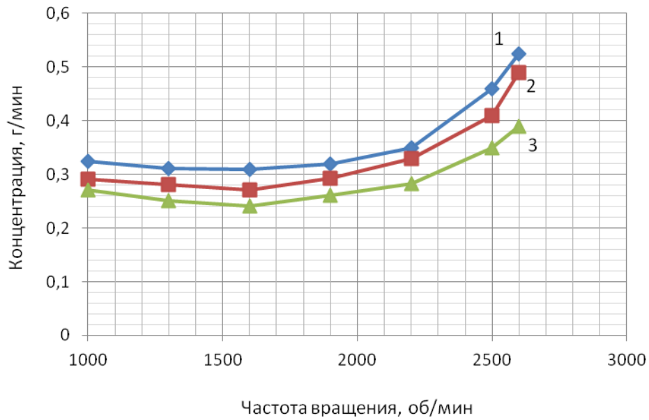
Рисунок 3.39 – Средние зависимости выбросов CO для двигателя Testor 6, установленного на автомобиле Iveco EuroCargo, мощностью 280 л.с. от частоты вращения коленчатого вала в режиме без нагрузки: 1 – базовая модель; 2 – при добавке 0,15% водорода к топливной смеси; 3 – при добавке 0,25% водорода к топливной смеси
