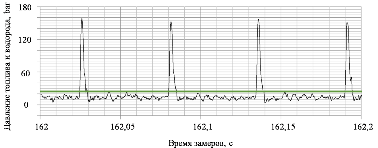
Рисунок 3.9 – Диаграмма впрыска топлива в ДВС специального автотранспорта при давлении подачи водородной примеси 0,2 МПа
