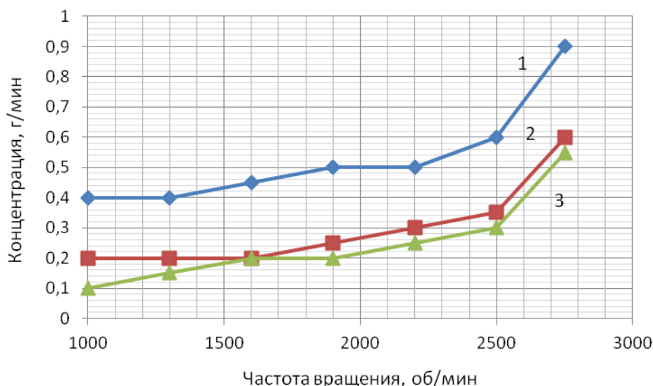
Рисунок 3.21 – Зависимости средних значений выбросов \text{SO}_2 для двигателя Tector 4, установленного на автомобиле Iveco EuroCargo, мощностью 160 л.с. без нагрузки от частоты вращения коленчатого вала: 1 – базовая модель; 2 – при добавке 0,15% водорода к топливной смеси; 3 – при добавке 0,25% водорода к топливной смеси
