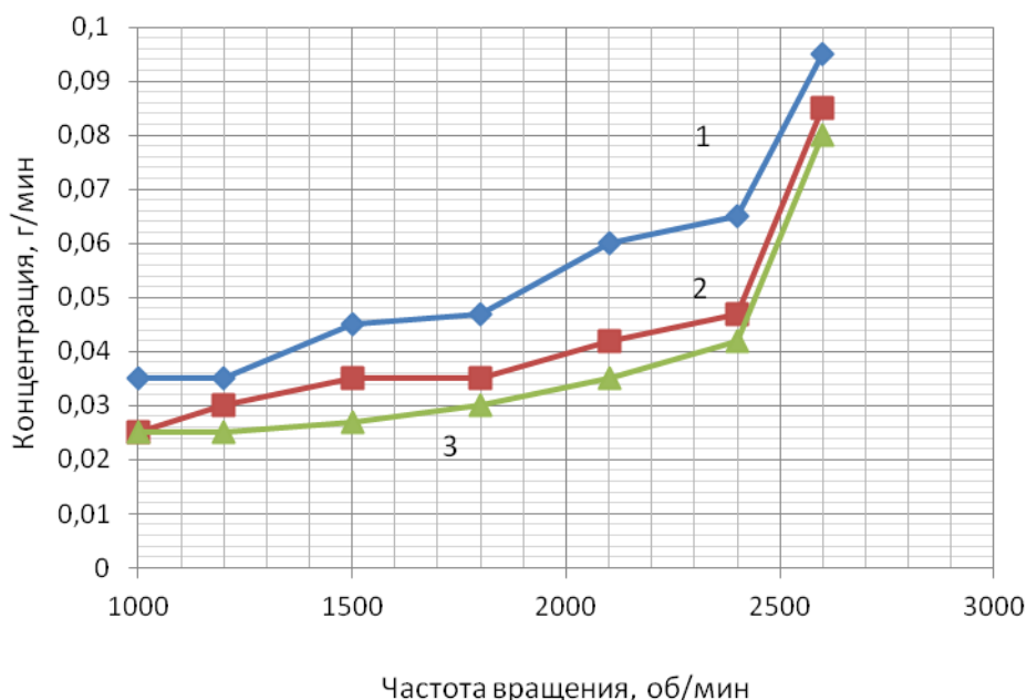
Рисунок 3.20 – Зависимости средних значений выбросов HC для двигателя Testor 4, установленного на автомобиле Iveco EuroCargo, мощностью 160 л.с. под нагрузкой от частоты вращения коленчатого вала: 1 – базовая модель; 2 – при добавке 0,15% водорода к топливной смеси; 3 – при добавке 0,25% водорода к топливной смеси
