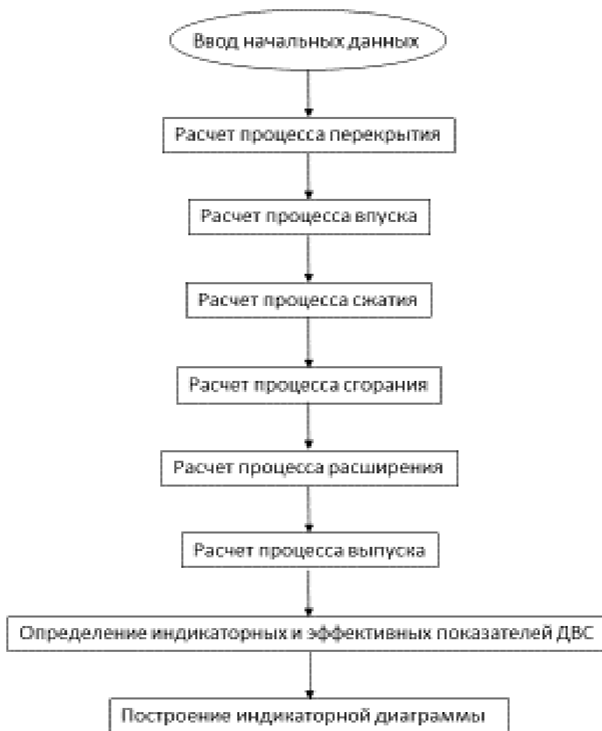
Рисунок 2.1 – Блок-схема математического моделирования рабочего процесса ДВС, работающего на совмещенном цикле дизеля и примесей водорода методом объемного баланса
