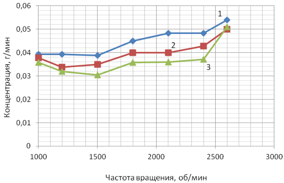
Рисунок 3.44 – Зависимости средних значений выбросов HC для двигателя Testor 6, установленного на автомобиле Iveco EuroCargo, мощностью 280 л.с. под нагрузкой от частоты вращения коленчатого вала: 1 – базовая модель; 2 – при добавке 0,15% водорода к топливной смеси; 3 – при добавке 0,25% водорода к топливной смеси
