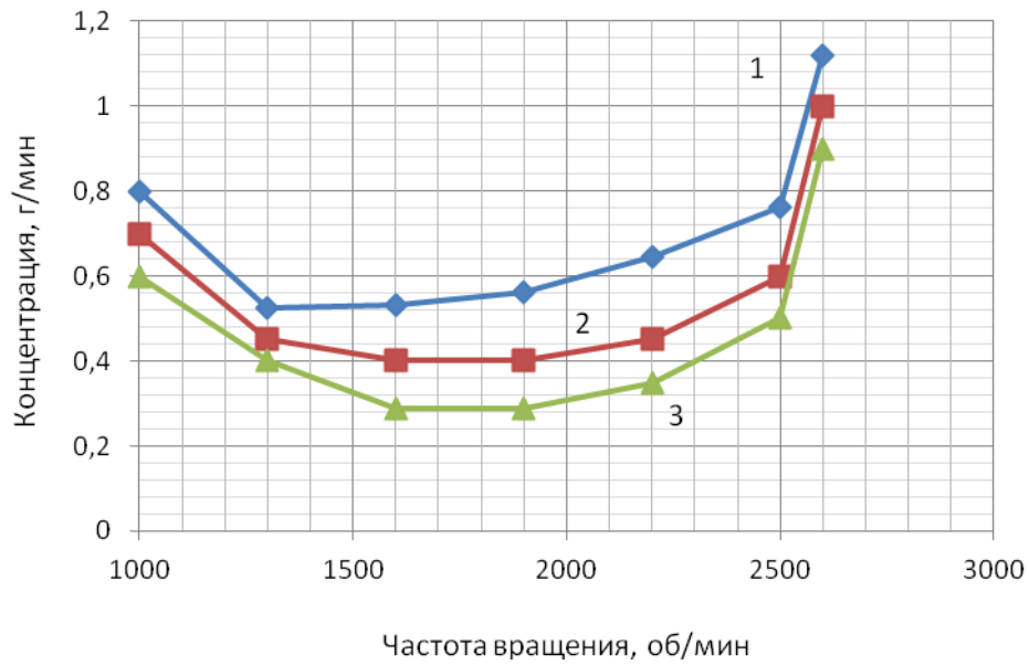
Рисунок 3.37 – Зависимости средних значений выбросов \text{SO}_2 для двигателя Tector 6, установленного на автомобиле Iveco EuroCargo, мощностью 220 л.с. без нагрузки от частоты вращения коленчатого вала: 1 – базовая модель; 2 – при добавке 0,15% водорода к топливной смеси; 3 – при добавке 0,25% водорода к топливной смеси
